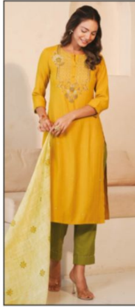
{1002}
